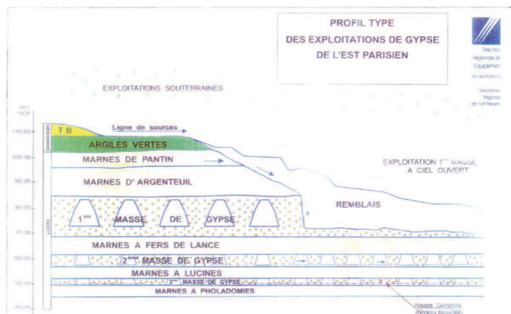
Figure 6: Profil type des exploitations de gypse de l'est parisien – Source : DRE Ile de France
