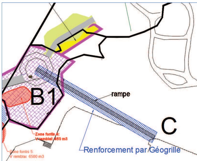
Figure 35: Renforcement par géogrille et remblais de la zone C - source: EGIS
